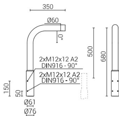
WR-8B/1/0,35/0
