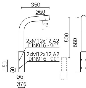
WR-8B/1/0,35/5
