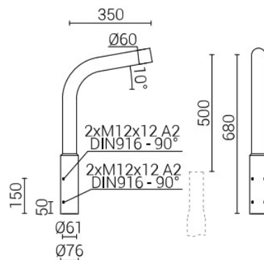
WR-8B/1/0,35/10
