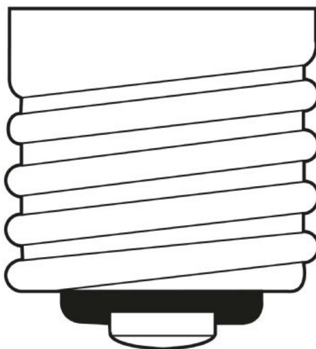
E40 IEC 7004-24 DIN 49625
