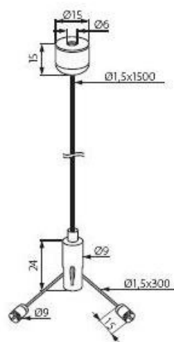
ROPE-NT 150
