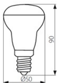
SIGO R50 LED E14-WW
