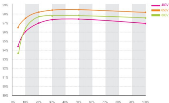
Growatt 6000TL3-S wydajność
