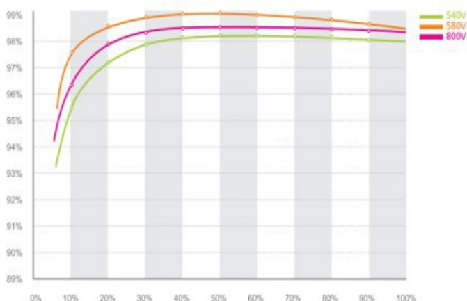
Growatt 17000TL3-S wydajność
